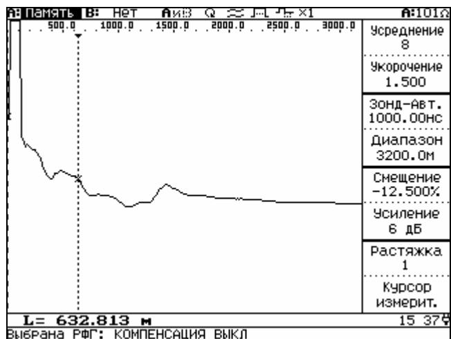
Без компенсации
